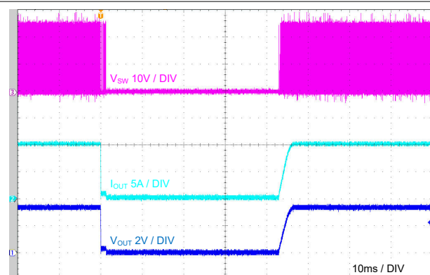
図 7-28. Load Transient, 0A to 5A
