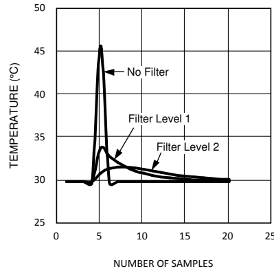
図 6-6. デジタル フィルタのインパルス応答
