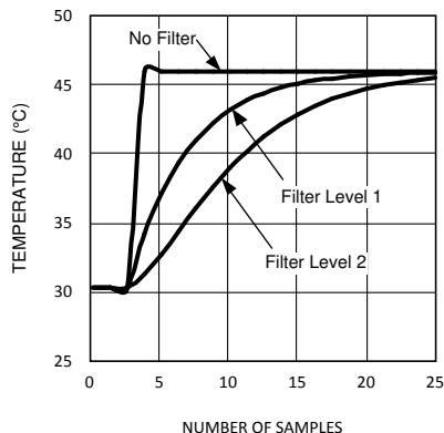
図 6-5. デジタルフィルタのステップ応答
