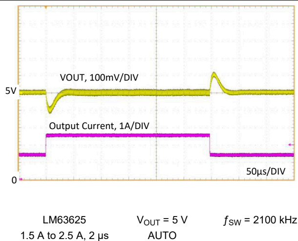
図 8-32. Load Transient
