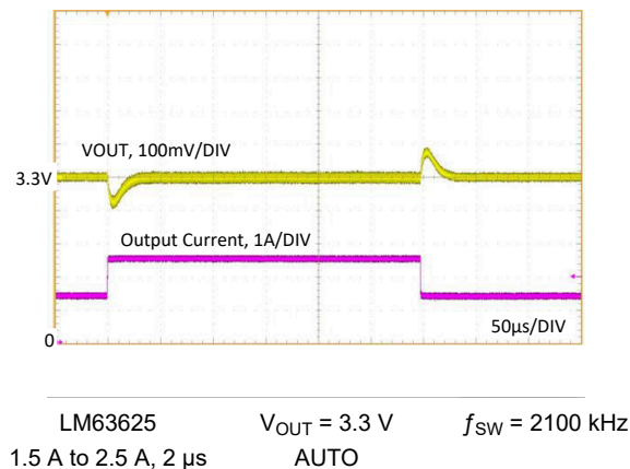
図 8-30. Load Transient
