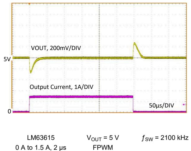
図 8-29. Load Transient
