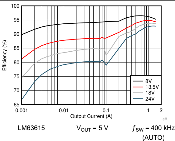
図 8-10. Efficiency
