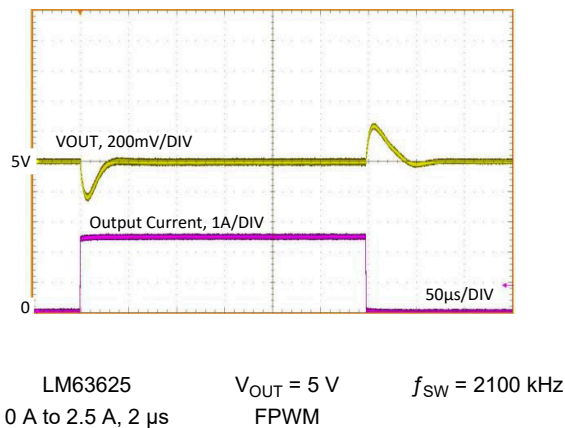
図 8-28. Load Transient
