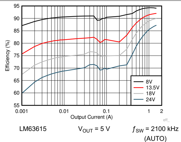
図 8-11. Efficiency
