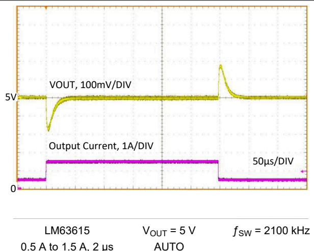
図 8-33. Load Transient
