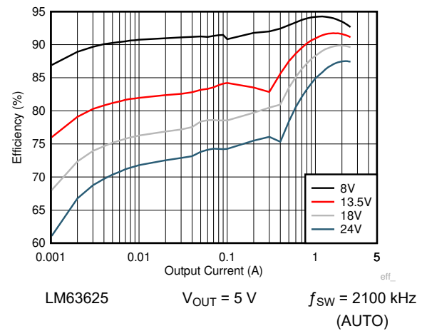
図 8-9. Efficiency
