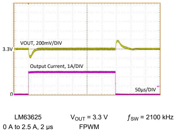
図 8-26. Load Transient
