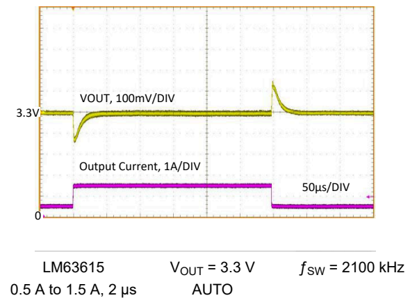
図 8-31. Load Transient
