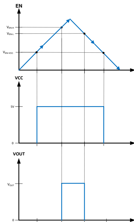
図 7-2. Precision Enable Behavior
