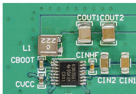
代表的なソリューション例: I_{\text{OUT}} = 2.5\text{A} 、 f_{\text{SW}} = 2200\text{kHz}
