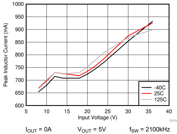
図 6-3. LM63625 の I_{PEAK-MIN}
