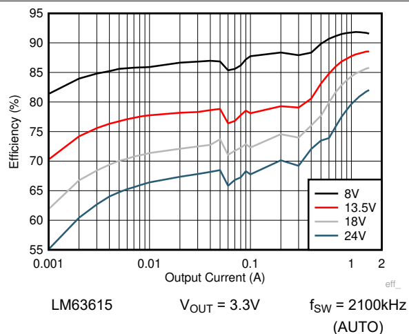
図 8-15. 効率
