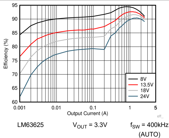
図 8-12. 効率
