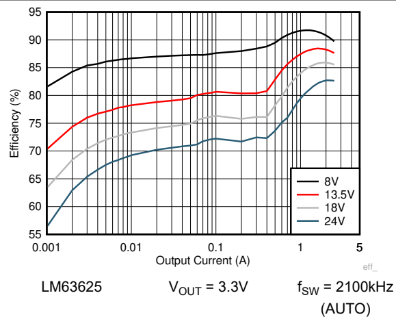
図 8-13. 効率
