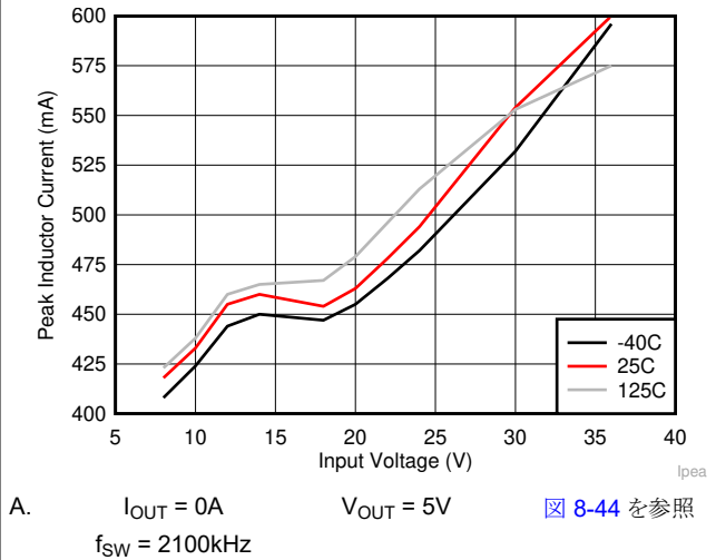
図 6-4. LM63615 の I_{PEAK-MIN}
