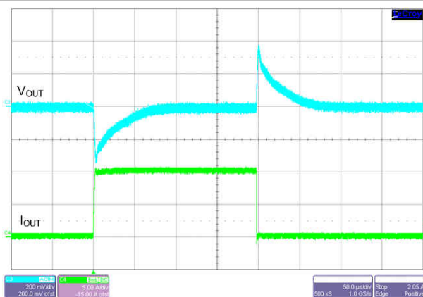
图 9-38. Load Transient
