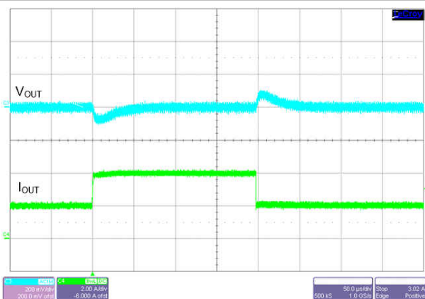
图 9-37. Load Transient
