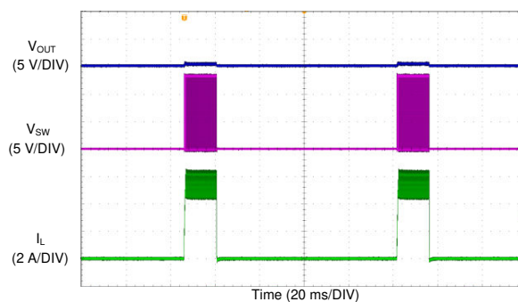
图 9-20. LM62435-Q1 Short Circuit Protection
