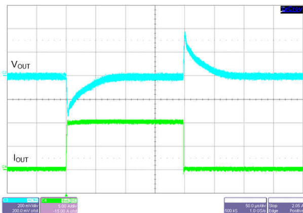
图 9-38. Load Transient
