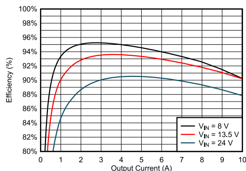
EVM の効率: V_{OUT} = 5V , F_{SW} = 2.2\text{MHz}
