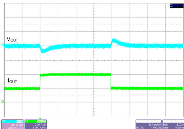
图 9-37. Load Transient
