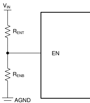
图 8-2. VIN UVLO Using the EN Pin
