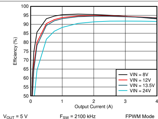
图 9-7. LM61440-Q1 Efficiency
