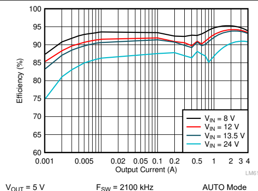
图 9-6. LM61440 Efficiency
