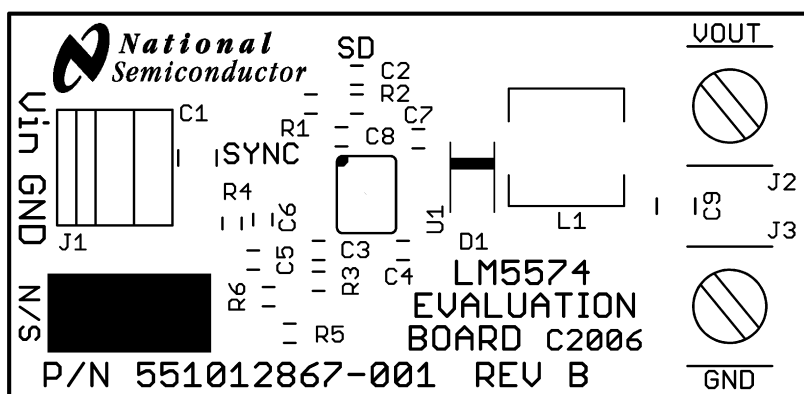
図 7-14. Silkscreen
