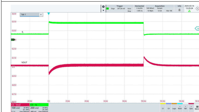
図 7-10. Load Regulation
