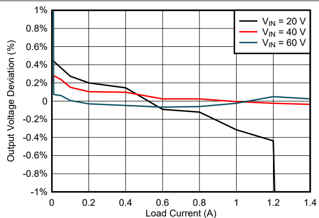
図 8-3. Load Regulation
