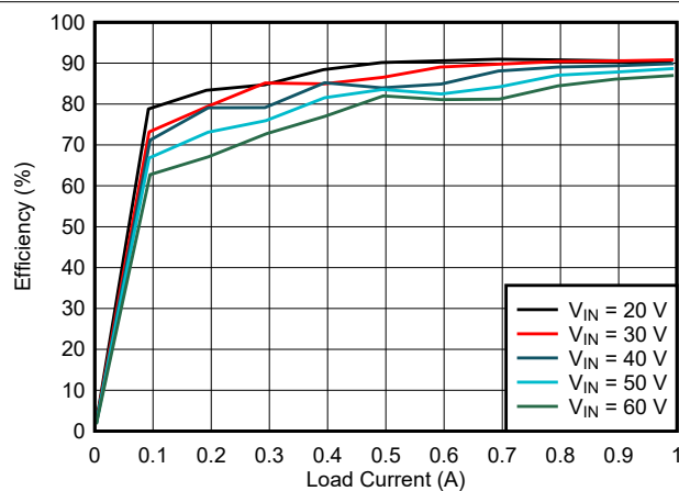
図 8-2. Efficiency
