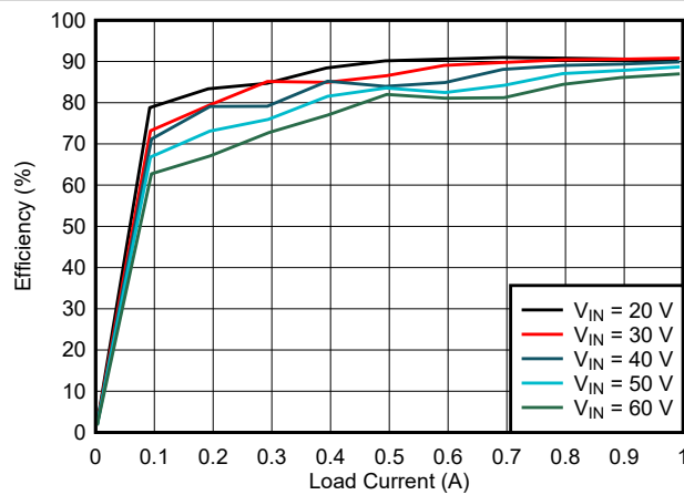
図 8-2. Efficiency
