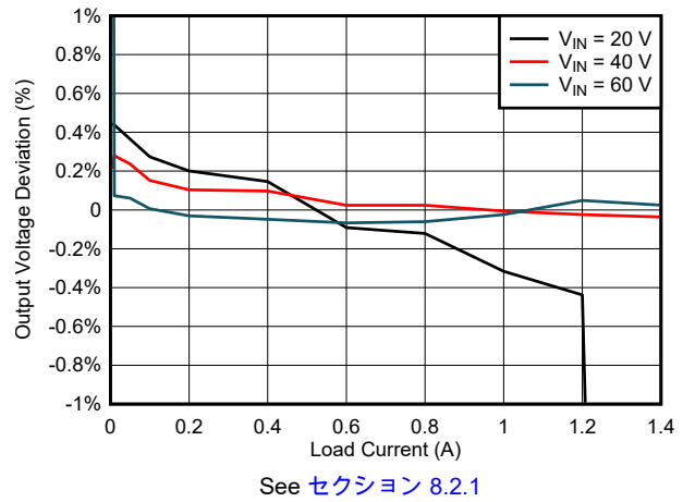
図 6-2. Output Voltage versus Load
