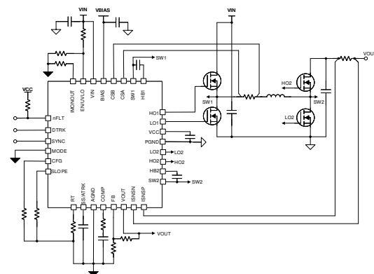
概略回路図
