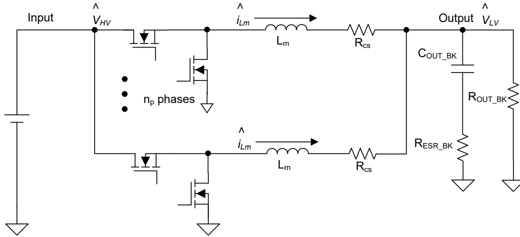
図 7-4. n_p phases system
