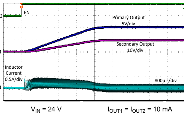
図 8-6. Light Load Start-Up from EN
