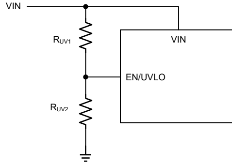
図 7-2. Input UVLO Connections
