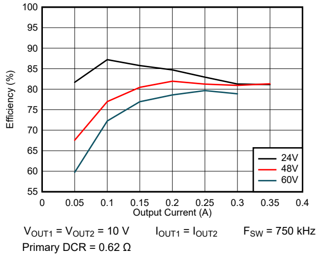
図 8-2. Efficiency
