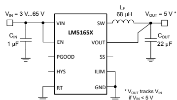
代表的な回路図、固定出力
