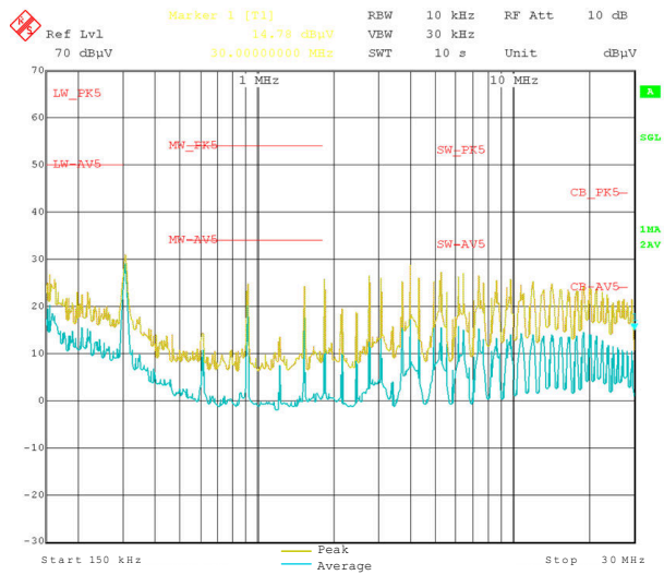
図 7-14. No-Load Switching
