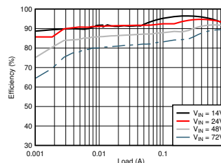
代表的なアプリケーションの効率、 V_{OUT} = 12V
