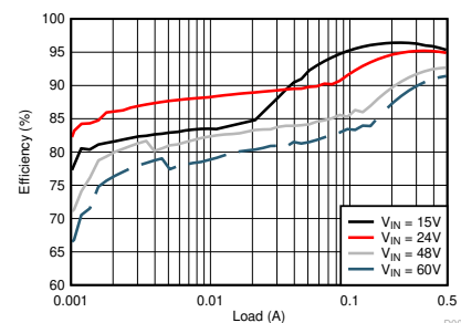
代表的なアプリケーションの効率、 V_{OUT} = 12\text{V}
