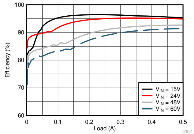
FIG 5-2. Conversion Efficiency (Linear Scale)
