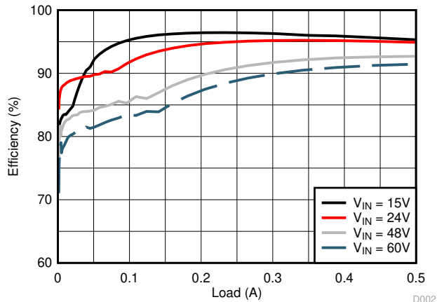
7-3. Conversion Efficiency (Linear Scale)
