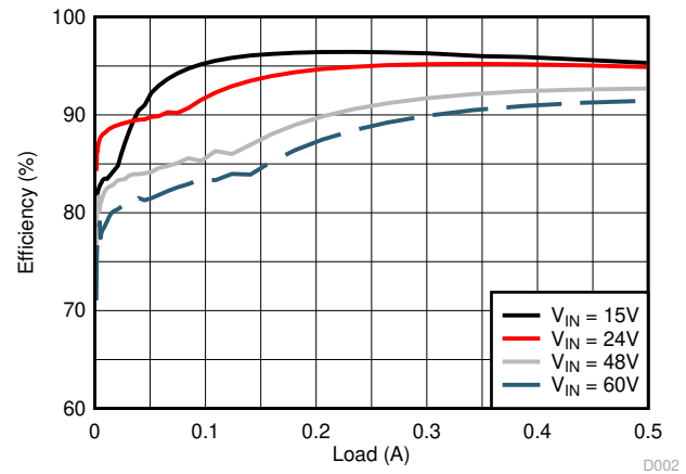
図 5-2. Conversion Efficiency (Linear Scale)
