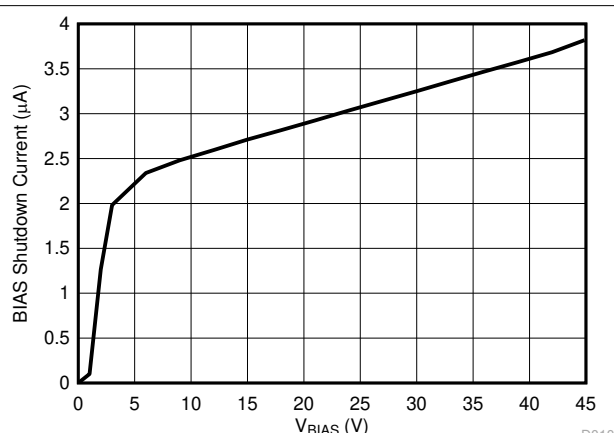
図 8-10. I_{\text{SHUTDOWN(BIAS)}} と V_{\text{BIAS}} との関係
