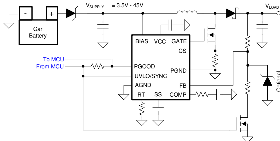
図 10-4. 代表的なスタート-ストップのアプリケーション
