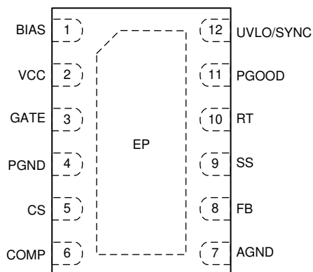
図 7-1. ウェットブル・フランク付き 12 ピン WSON DSS パッケージ (上面図)
