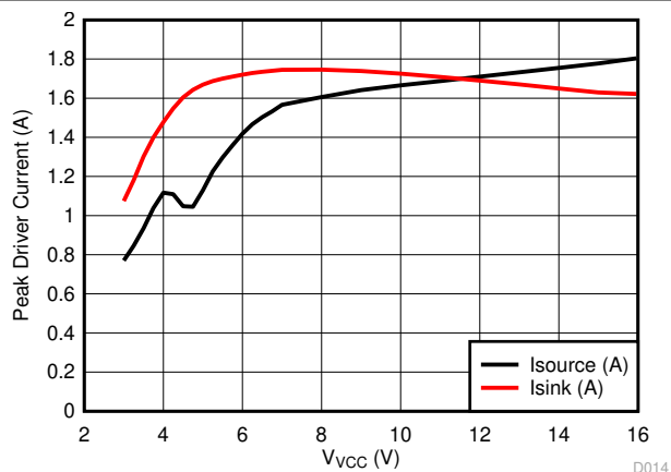
図 8-14. ピーク・ドライバ電流と V_{VCC} との関係
