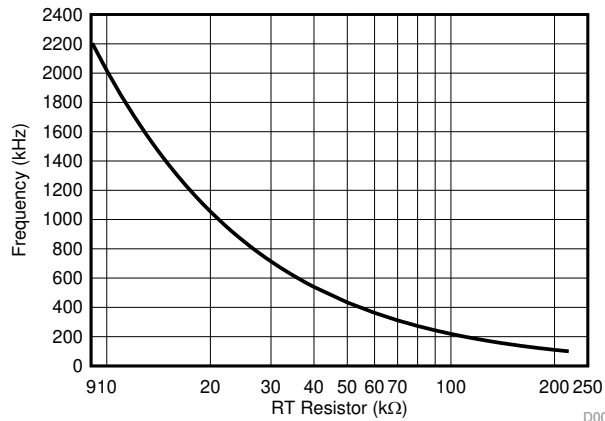
図 8-1. 周波数と RT 抵抗との関係
