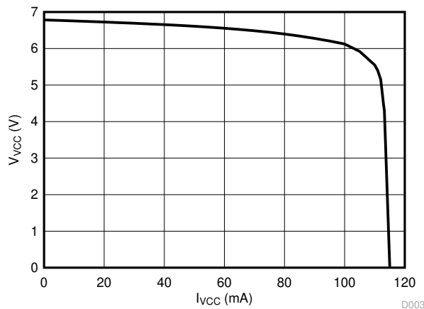
図 8-3. V VCC と I VCC との関係
