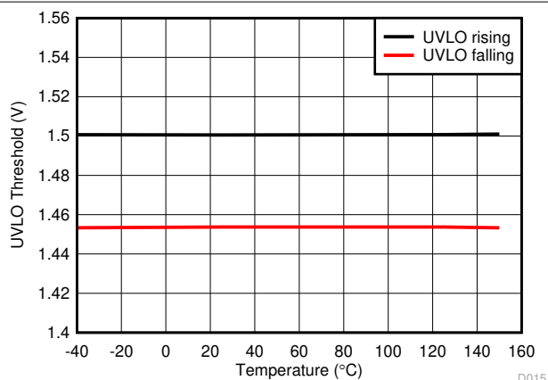
図 8-15. UVLO スレッシュホルドと温度との関係
