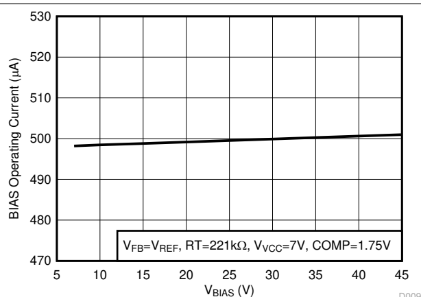
図 8-9. RT 電流を含む I_{\text{OPERATING(BIAS)}} と V_{\text{BIAS}} との関係
