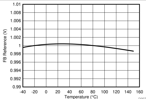
図 8-7. FB リファレンス電圧と温度との関係
