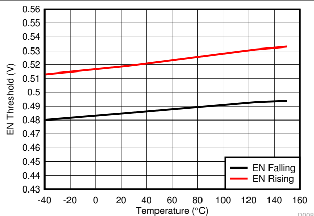
図 8-8. EN スレッシュホールドと温度との関係
