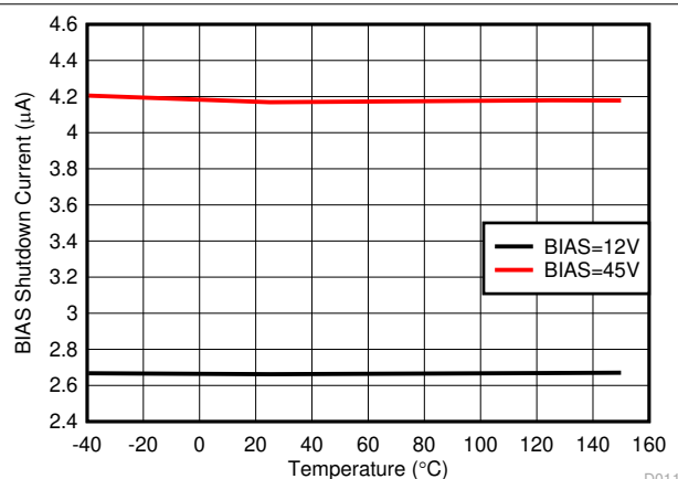
図 8-11. I_{\text{SHUTDOWN}} と温度との関係
