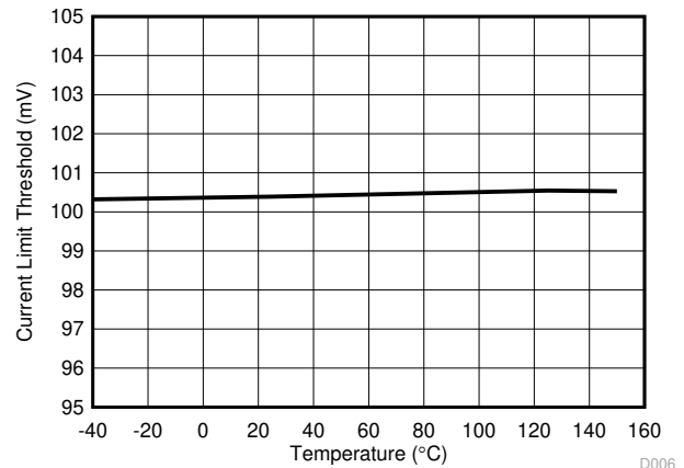
図 8-6. 電流制限スレッシュホールドと温度との関係
