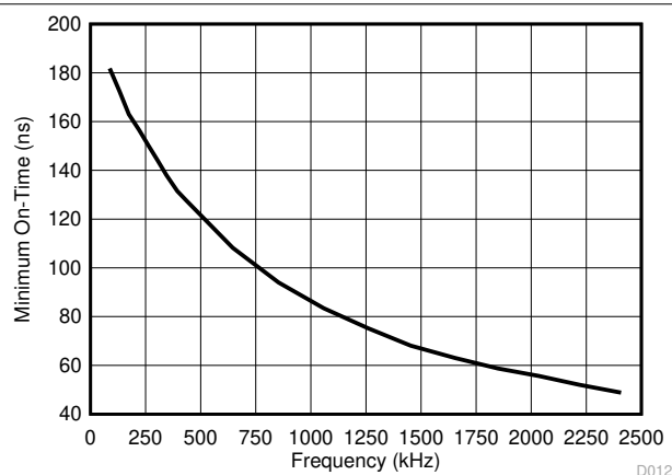
図 8-12. t_{\text{ON(MIN)}} と周波数との関係
