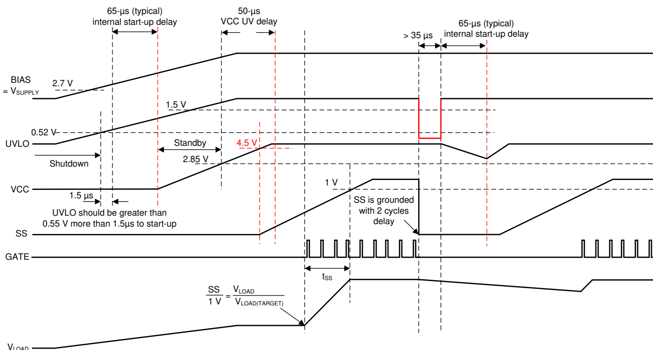
図 9-3. 昇圧スタートアップ波形ケース 2: VCC > 4.5V のときのスタートアップ、スタートアップ後の EN トグル
