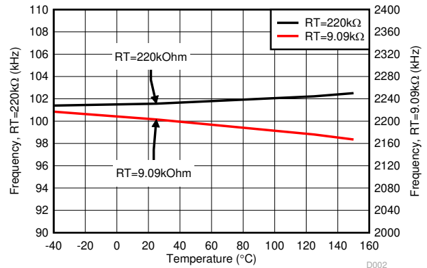
図 8-2. 周波数と温度との関係
