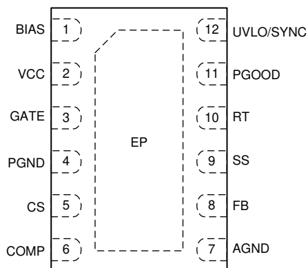
図 7-1. 12 ピン WSON DSS パッケージ (上面図)
