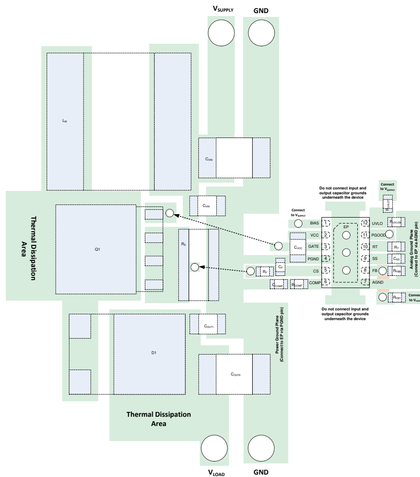
図 10-15. PCB のレイアウト例 1
