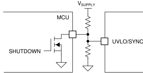
図 9-10. UVLO とシャットダウン
