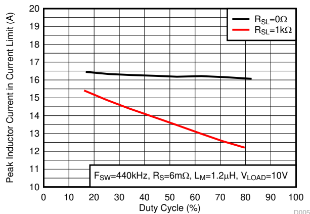
図 8-5. ピーク電流制限とデューティ・サイクルとの関係
