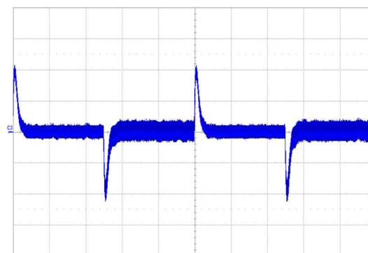
图 9-5. Load Transient
