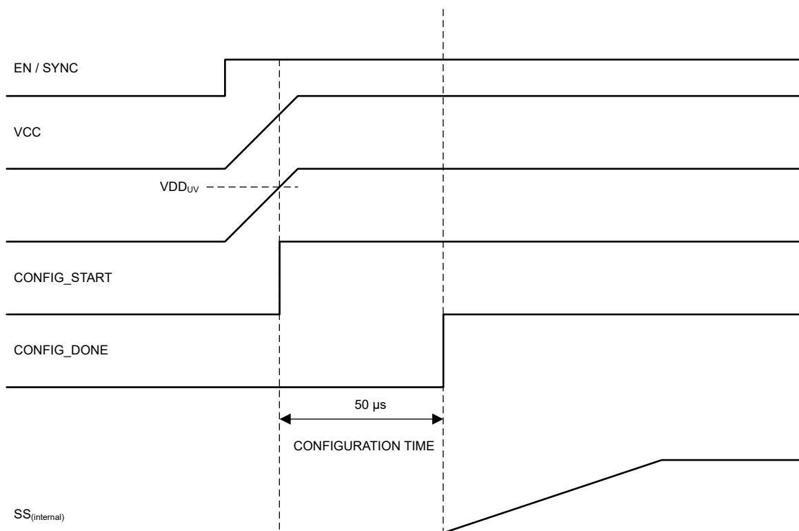
図 8-6. Configuration Timing
