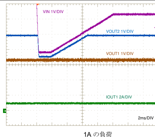
図 10-10. V_{IN} = 3.8V までのコールド・クランク応答
