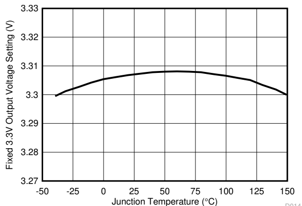
図 8-10. 固定 3.3V 出力電圧 (VOUT1) と温度との関係
