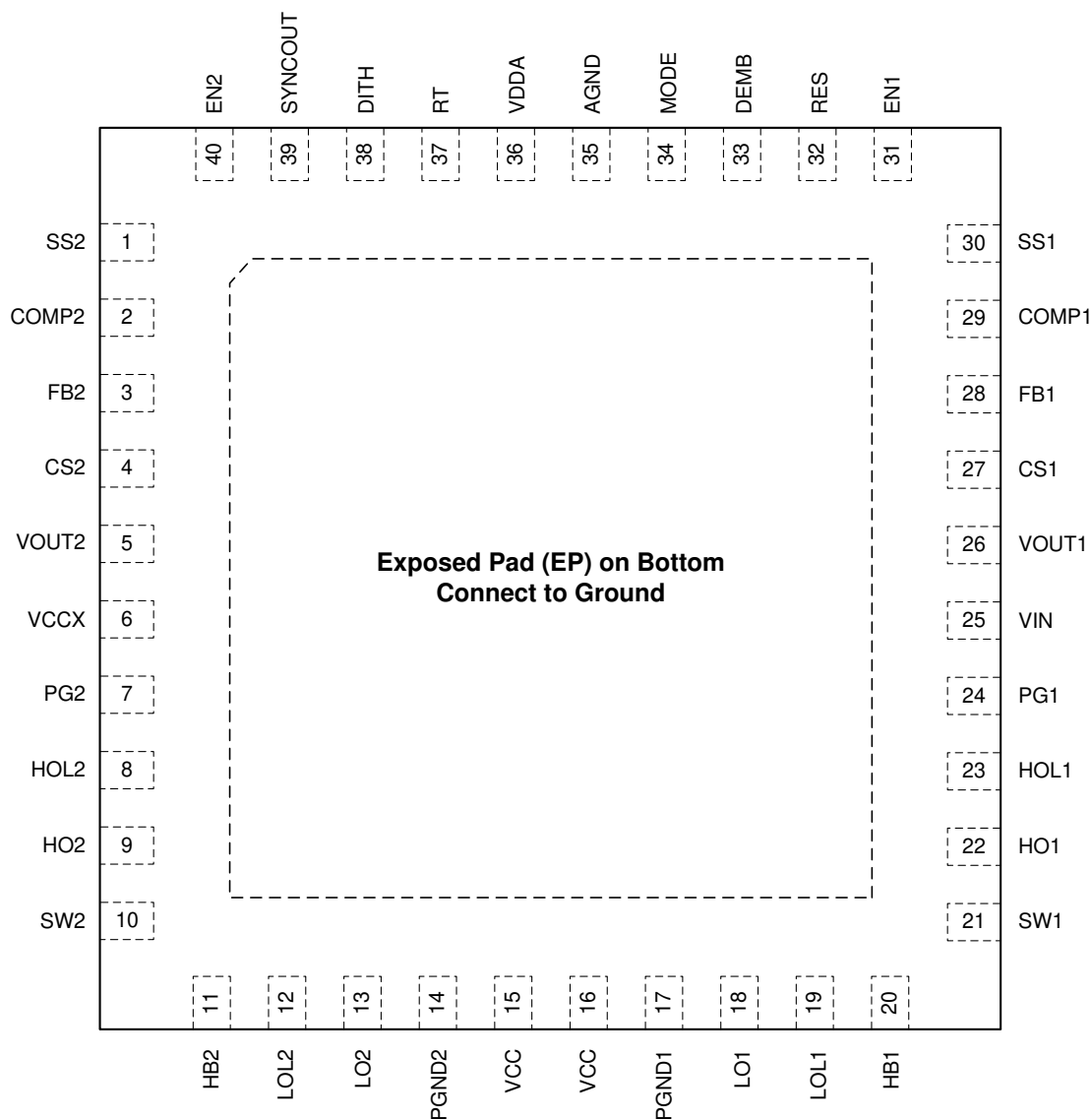
図 7-1. パッケージ (上面図)
