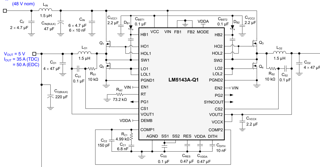
図 10-24. アプリケーション回路 3、LM5143A-Q1 2 相降圧レギュレータを 300kHz で使用
