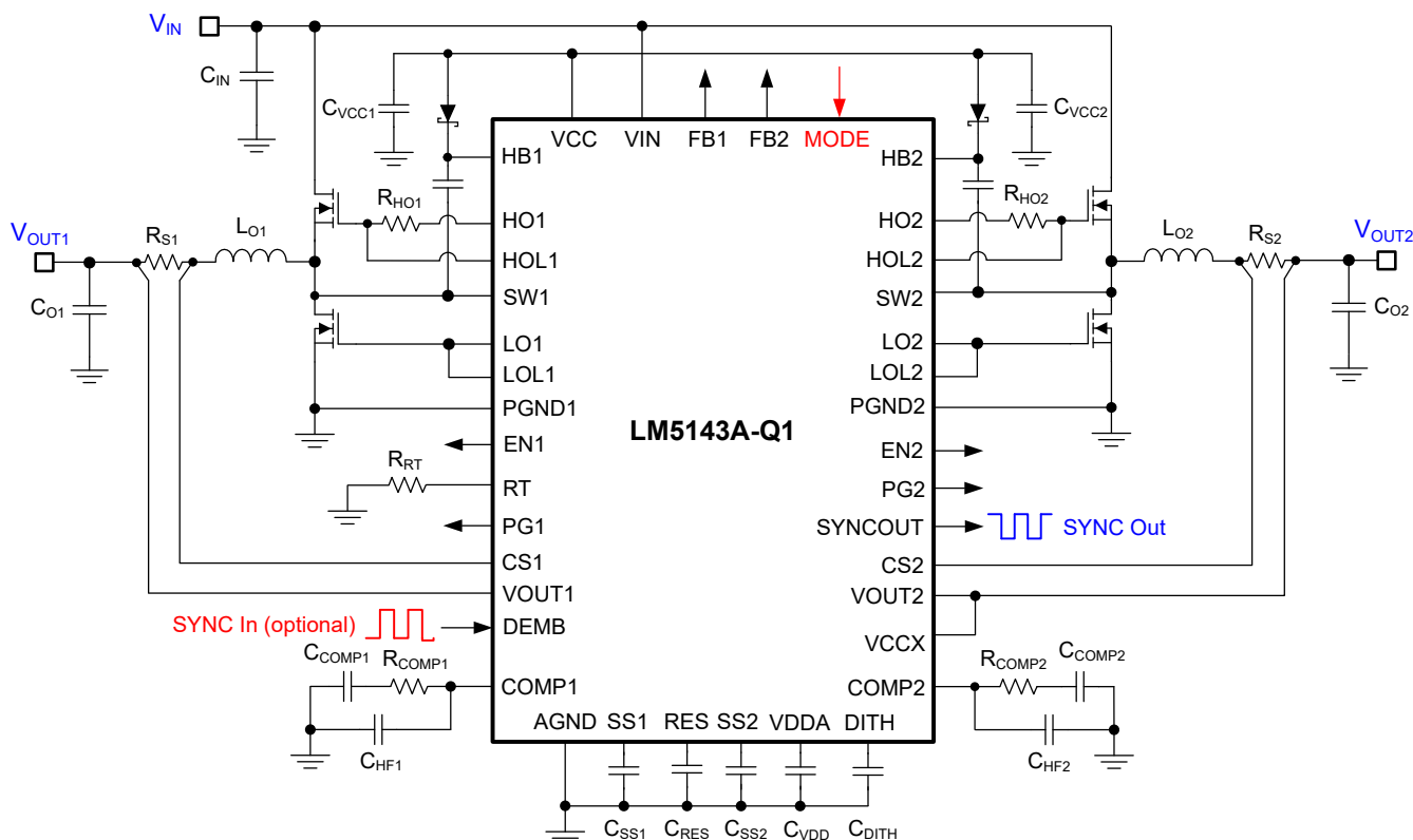
図 9-1. 入力電圧範囲 3.5V～65V のデュアル出力レギュレータの回路図
