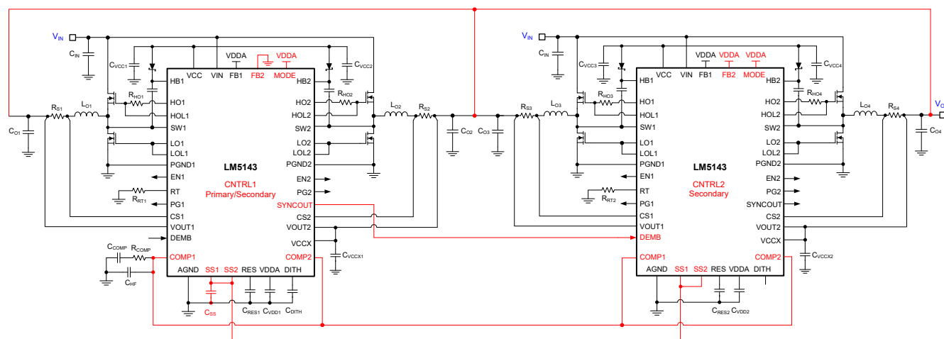
図 9-10. 単一出力インターリーブ動作に構成された多相レギュレータの回路図
