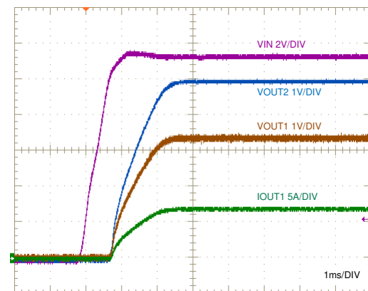
図 10-4 を参照してください。 図 8-4. スタートアップ特性
