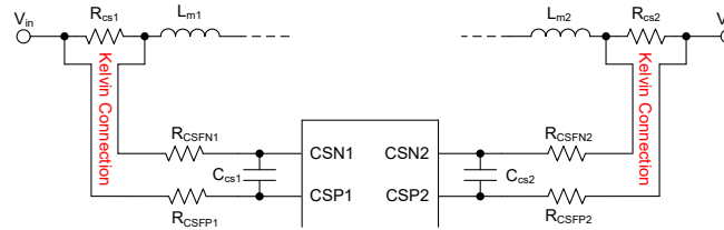
図 8-5. 電流センス フィルタ
