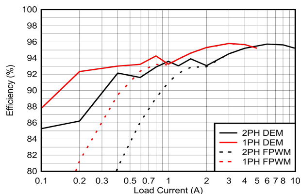
図 8-11. 効率と出力電流との関係、 V_{IN} = 14.4V 、 V_{OUT} = 45V
