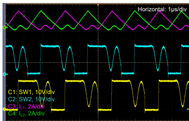
図 8-13. V_{IN} = 14.4V 、 V_{OUT} = 24V 、DEM、 I_{LOAD} = 1A
