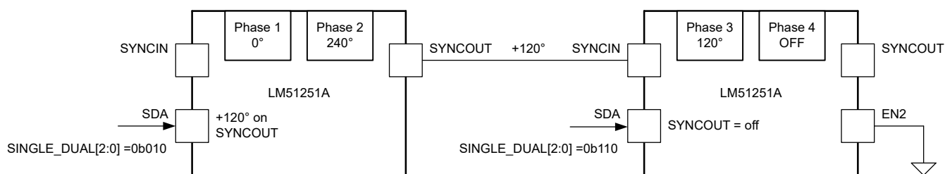
図 6-6. 3 相構成
