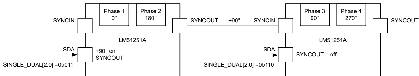
図 6-7. 4 相構成
