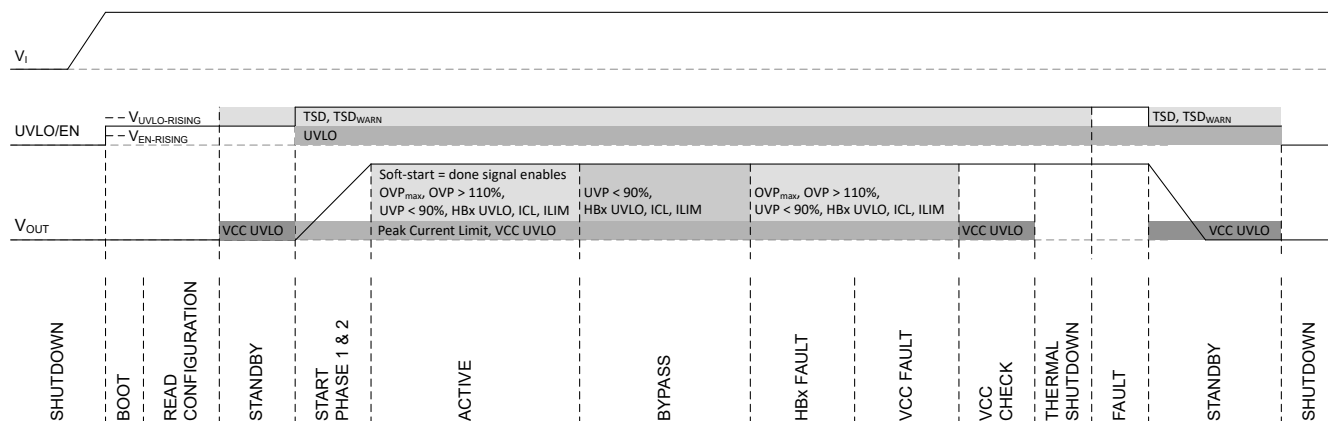
図 6-19. 保護素子
