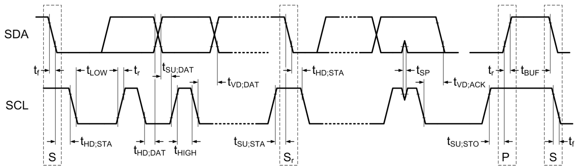
図 6-31. I 2 C データ送信タイミング
