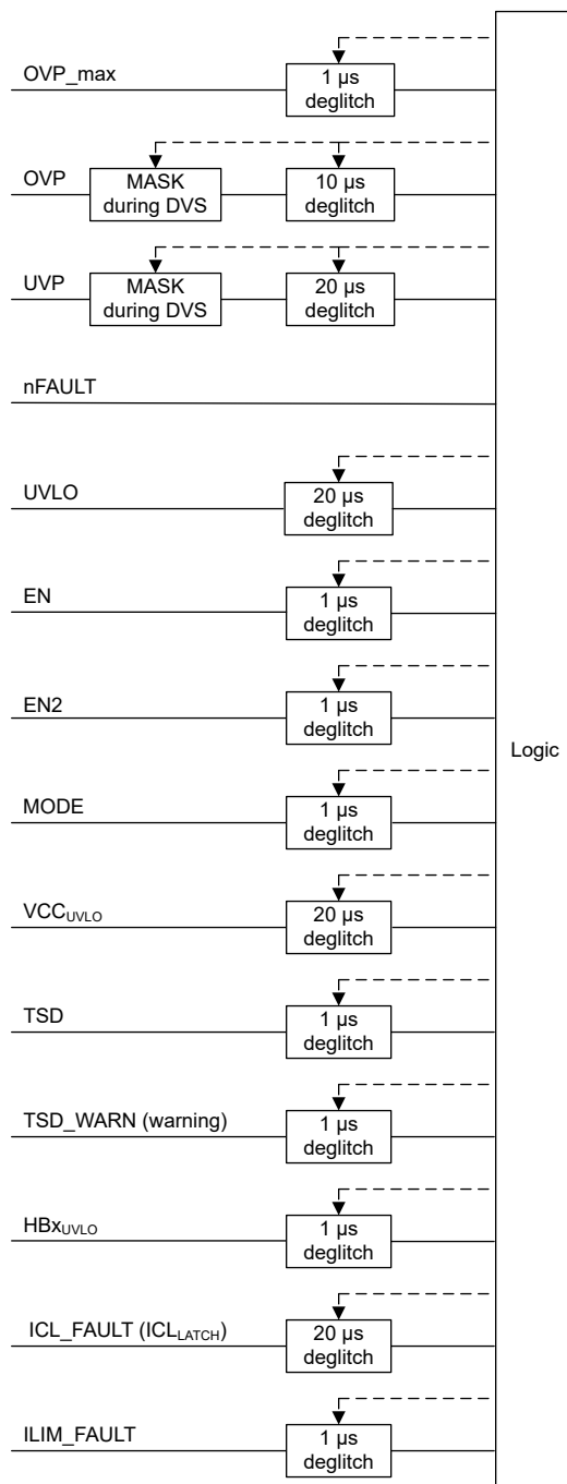
図 6-26. 信号のグリッチ除去
