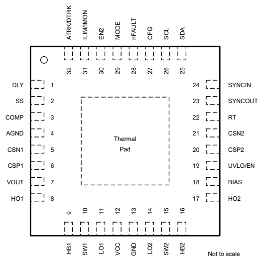
図 4-1. LM51251A-Q1 RHB パッケージ、32 ピン VQFN (上面図)
