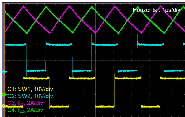
図 8-14. V_{IN} = 14.4V 、 V_{OUT} = 24V 、DEM、 I_{LOAD} = 15A
