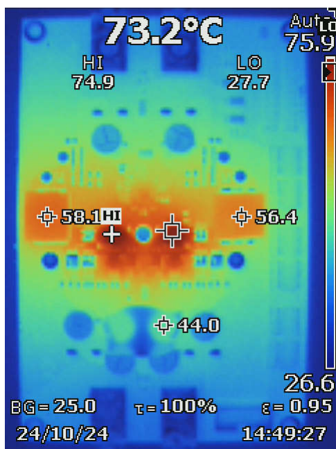
図 8-20. V_{IN} = 14.4V 、 V_{OUT} = 24V 、 P_{OUT} = 300W 、自然対流
