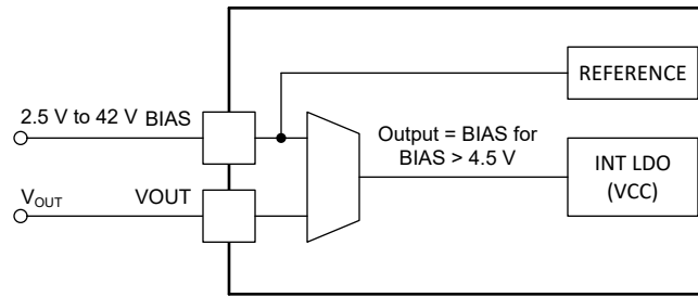
図 6-14. その場でのバイアス電源の選択
