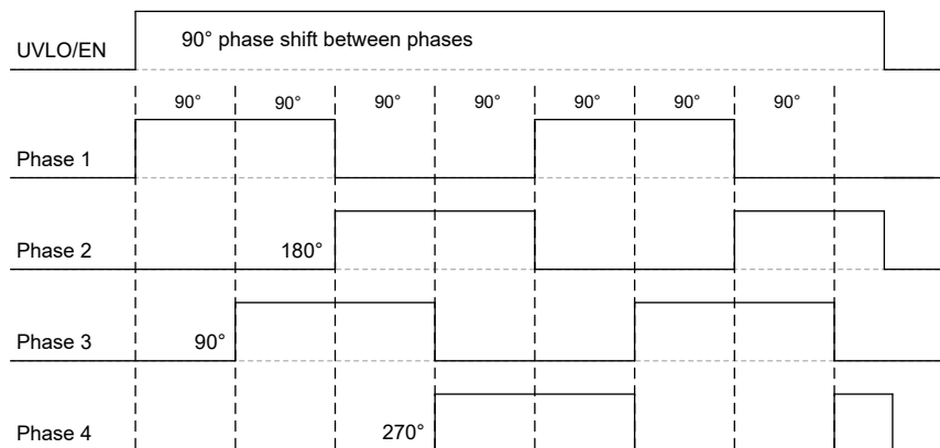
図 6-5. 2 つのデバイスの 4 相動作
