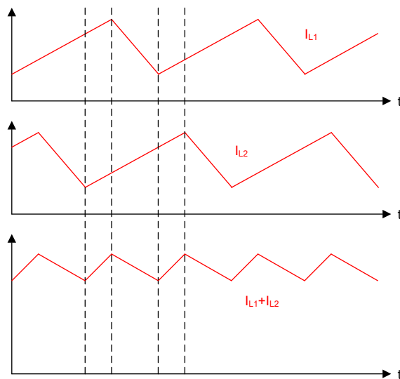
図 8-9. 正規化入力コンデンサ RMS リップル電流
