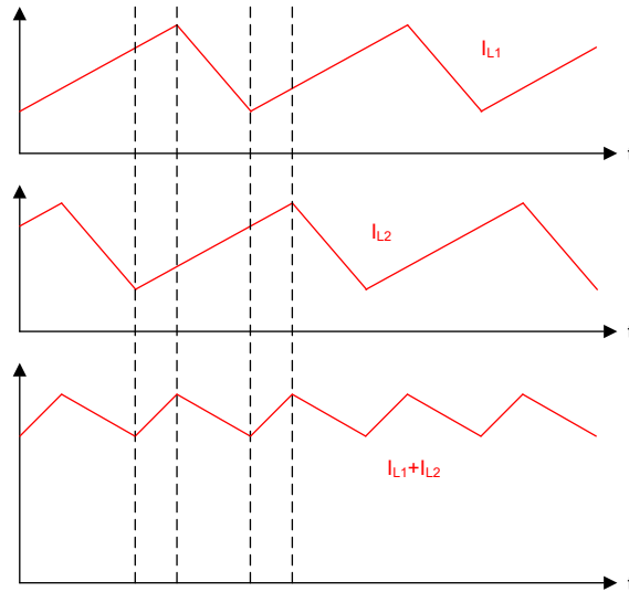
図 8-4. デュアル位相インターリーブにより、入力電流リップルが低減
