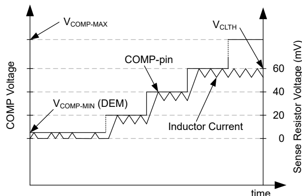
図 6-22. COMP ピンおよびセンス抵抗電圧によるスイッチ電流の制限 (DEM)
