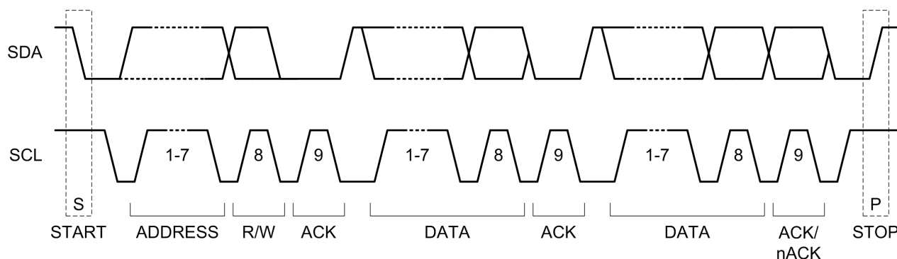
図 6-30. I 2 C スタート/ストップ/アクノリッジのプロトコル
