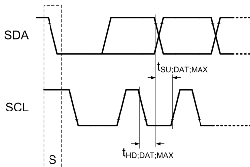
図 6-32. 最大の立ち上がり/立ち下がり時間の I 2 C データ送信タイミング
