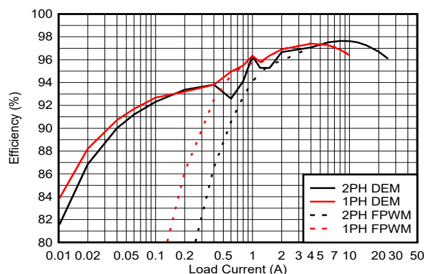
図 8-10. 効率と出力電流との関係、 V_{IN} = 14.4V 、 V_{OUT} = 24V
