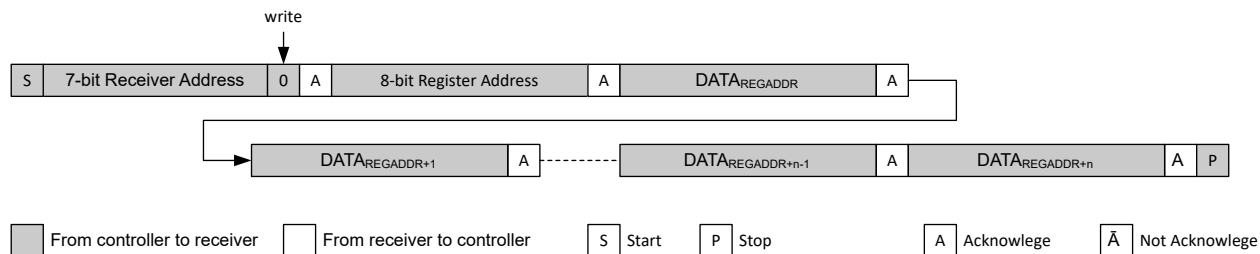
図 6-36. 定義されたレジスタ アドレスから開始されるシーケンシャル WRITE
