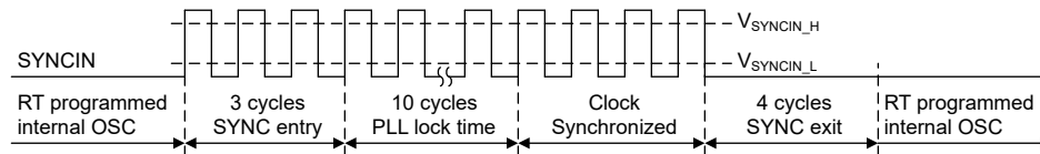
図 6-10. クロックの同期
