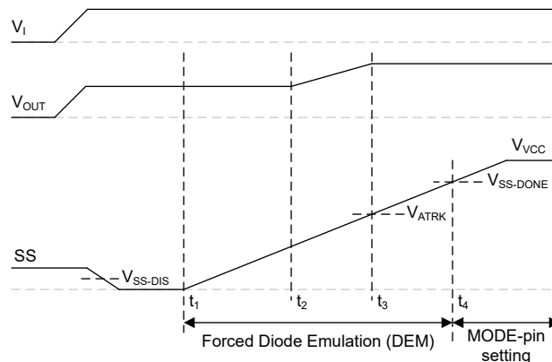
図 6-15. ソフト スタート
