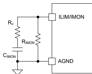
図 8-7. ILIM/IMON ピンの構成
