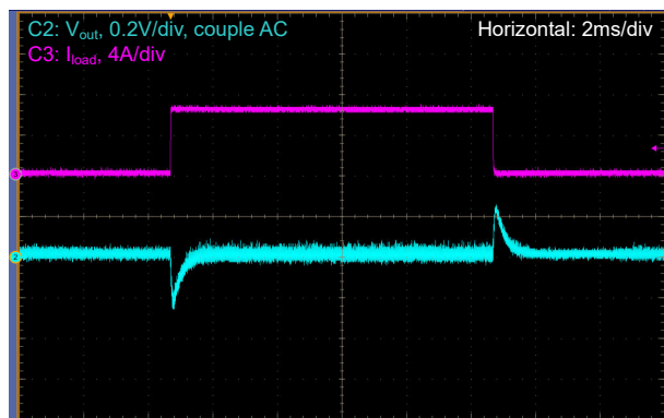
図 8-15. 負荷過渡、 V_{IN} = 14.4V 、 V_{OUT} = 24V 、FPWM、 I_{LOAD} = 0A \sim 6.25A ( 1A/\mu s )
