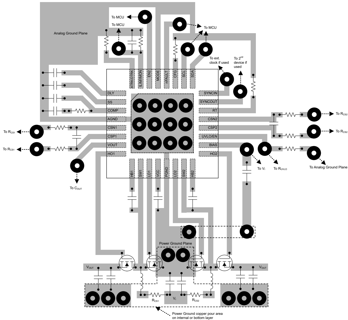
図 8-22. レイアウト例
