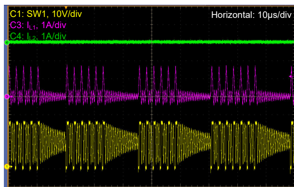
図 8-12. V_{IN} = 14.4V 、 V_{OUT} = 24V 、DEM、 I_{LOAD} = 0.1A
