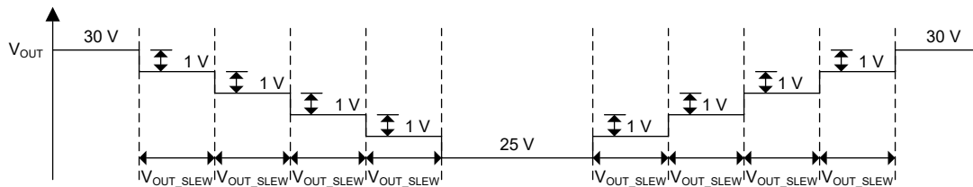
図 6-28. V_{OUT} プログラミングの例：30V から 25V へ、さらに 30V へ
