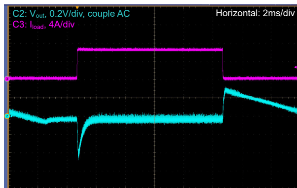
図 8-16. 負荷過渡、 V_{IN} = 14.4V 、 V_{OUT} = 24V 、DEM、 I_{LOAD} = 0A \sim 6.25A ( 1A/\mu s )
