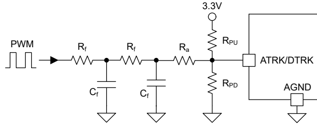
図 8-6. 2 段 RC フィルタから ATRK/DTRK へ
