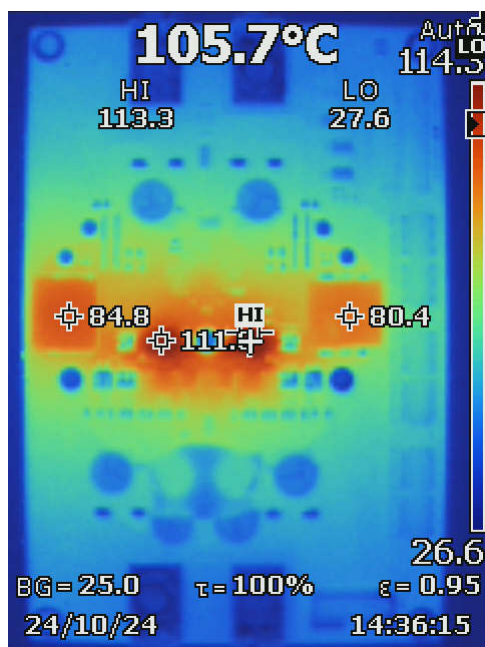
図 8-21. V_{IN} = 14.4V 、 V_{OUT} = 45V 、 P_{OUT} = 300W 、自然対流
