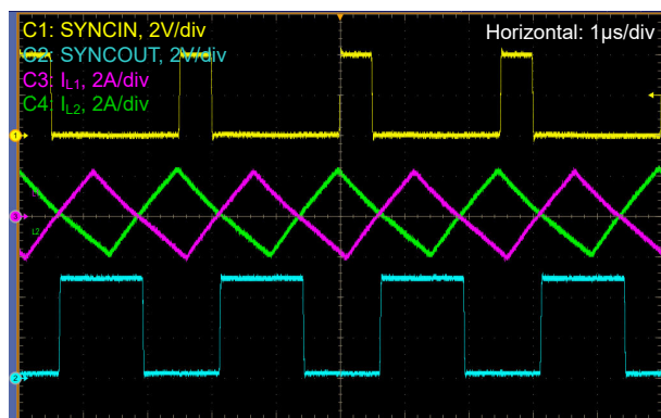
図 8-17. V_{IN} = 14.4V 、 V_{OUT} = 24V 、FPWM、 I_{LOAD} = 0A 、CFG2 = レベル 13
