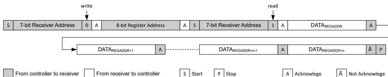
図 6-34. 定義されたレジスタ アドレスから開始されるシーケンシャル READ
