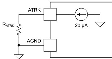
図 6-16. 抵抗による V OUT のプログラミング
