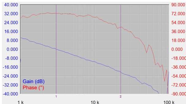
図 8-19. ボード線図、 V_{IN} = 14.4V 、 V_{OUT} = 40V 、 I_{OUT} = 10A (平均電流ループ無効化)
