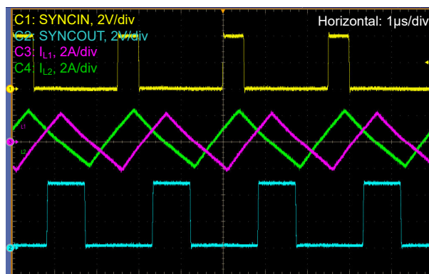
図 8-18. V_{IN} = 14.4V 、 V_{OUT} = 24V 、FPWM、 I_{LOAD} = 0A 、CFG2 = レベル 11
