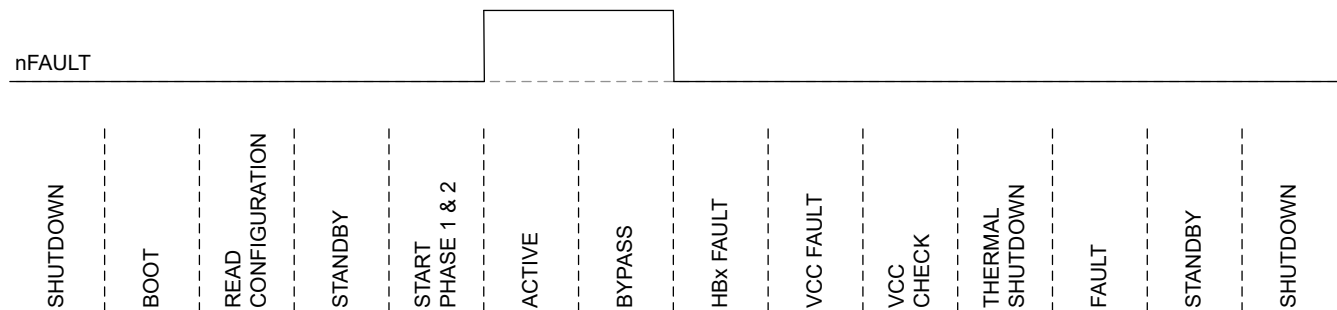
図 6-20. すべてのデバイス状態の nFAULT ステータス
