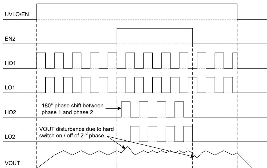
図 6-3. の 2 相動作
