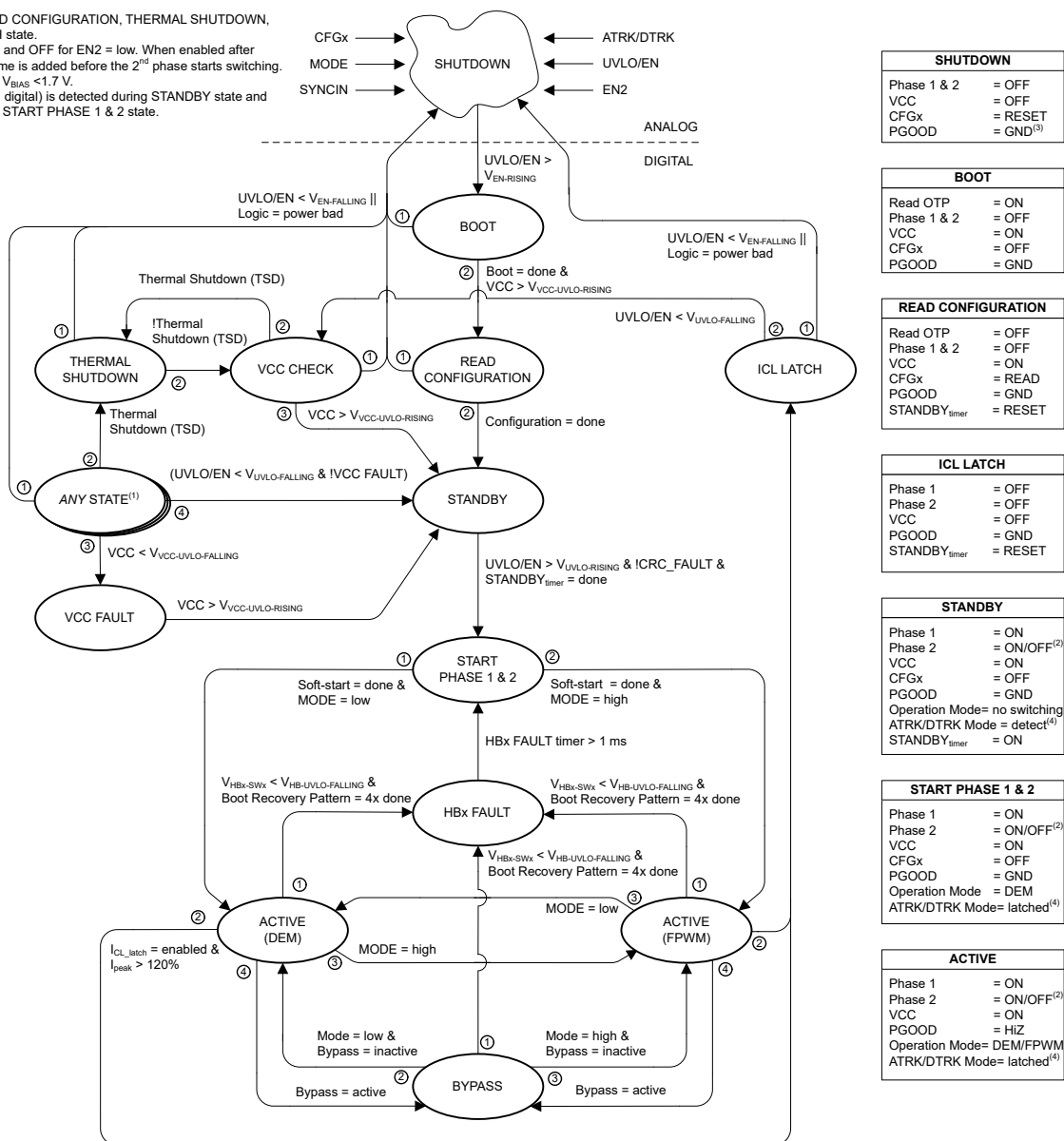
図 6-19. 機能状態図
