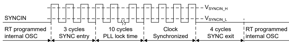
図 6-3. クロックの同期
