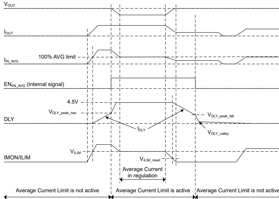
図 6-15. 平均電流制限
