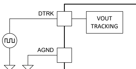
図 6-10. デジタル信号による V_{OUT} のトラッキング
