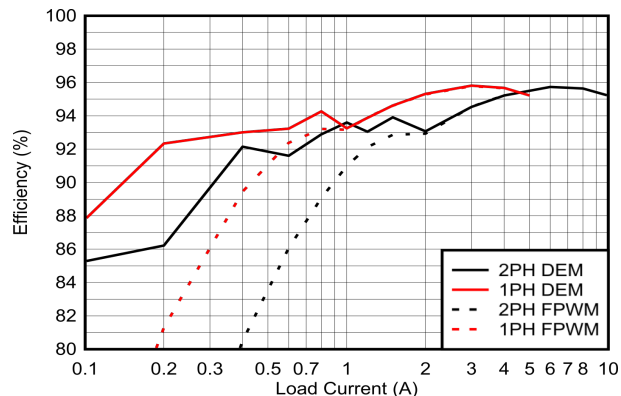
図 7-13. 効率と出力電流との関係、 V_{in} = 14.4V 、 V_{out} = 45V
