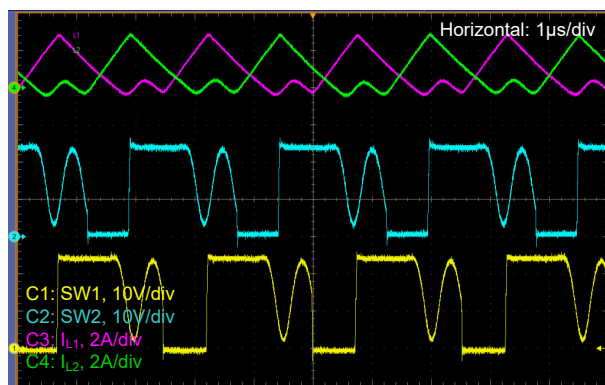
図 7-15. V_{in} = 14.4V 、 V_{out} = 24V 、DEM、 I_{load} = 1A
