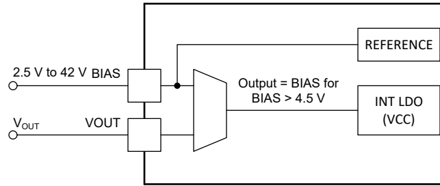
図 6-6. その場でのバイアス電源の選択
