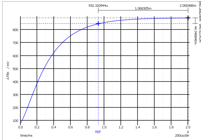
図 7-8. ATRK/DTRK の立ち上がり時間
