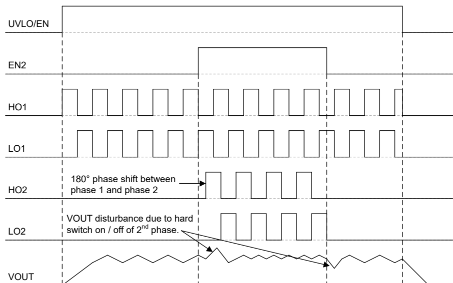
図 6-2. の 2 相動作
