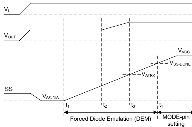
図 6-7. ソフト スタート
