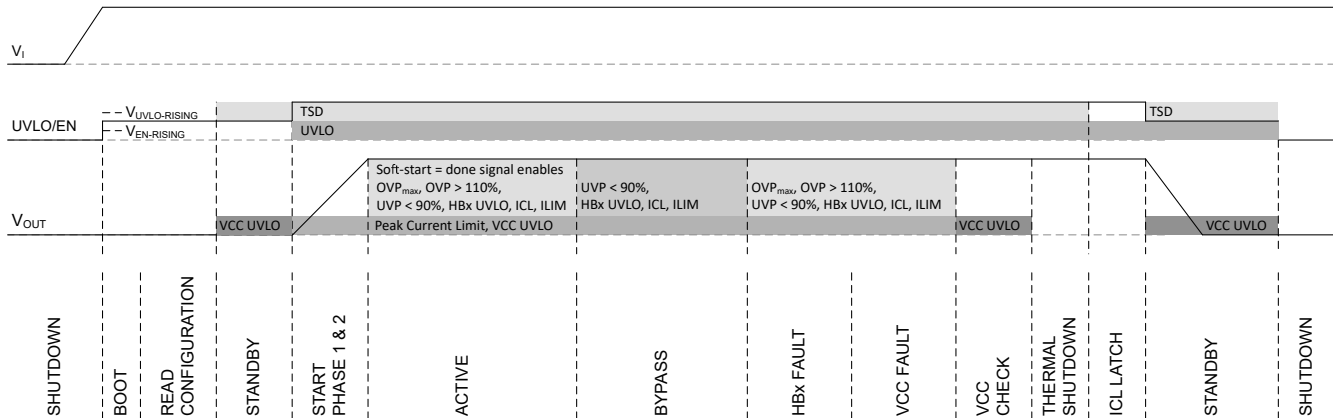
図 6-11. 保護素子
