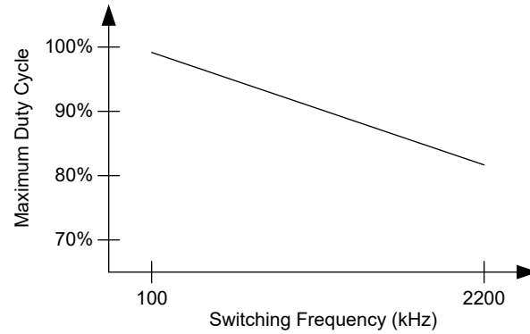
図 6-16. スイッチング周波数と最大デューティ サイクルとの関係
