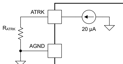
図 6-8. 抵抗による V_{OUT} のプログラミング
