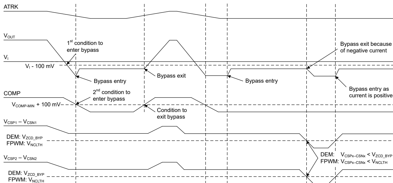
図 6-5. バイパス モードの開始、終了
