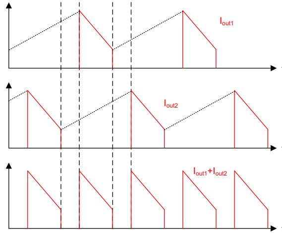
図 7-10. 正規化された出力コンデンサの RMS リップル電流
