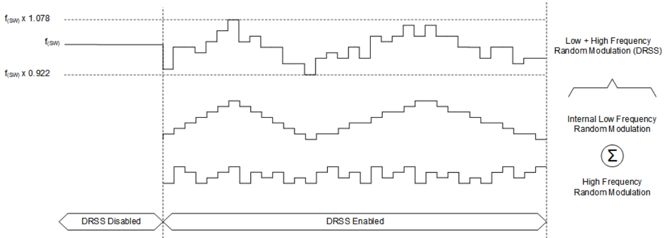
図 6-4. デュアル ランダム スペクトラム拡散
