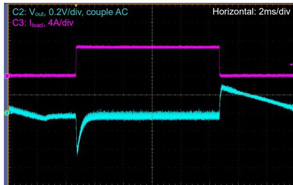
図 7-18. 負荷過渡応答、 V_{in} = 14.4V 、 V_{out} = 24V 、 DEM 、 I_{load} = 0A \sim 6.25A ( 1A/\mu s )
