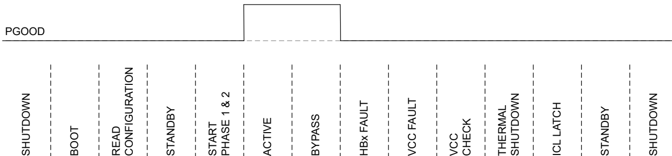
図 6-12. すべてのデバイス状態の PGOOD ステータス
