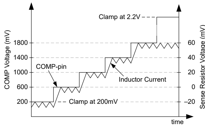
図 6-14. COMP ピンおよびセンス抵抗電圧スイッチ電流を制限します
