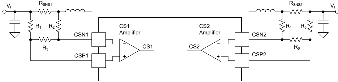
図 6-13. 追加の抵抗によりピーク制限を調整できます
