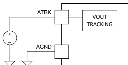
図 6-9. アナログ電圧による V_{OUT} のトラッキング
