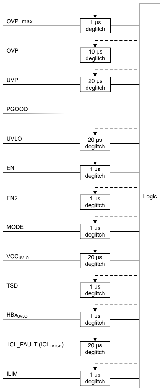
図 6-17. 信号のグリッチ除去
