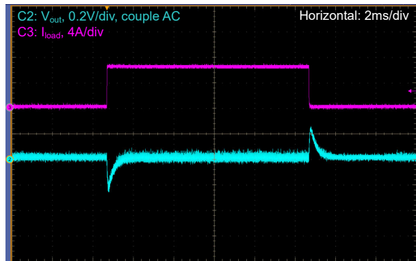
図 7-17. 負荷過渡応答、 V_{in} = 14.4V 、 V_{out} = 24V 、 FPWM 、 I_{load} = 0A \sim 6.25A ( 1A/\mu s )
