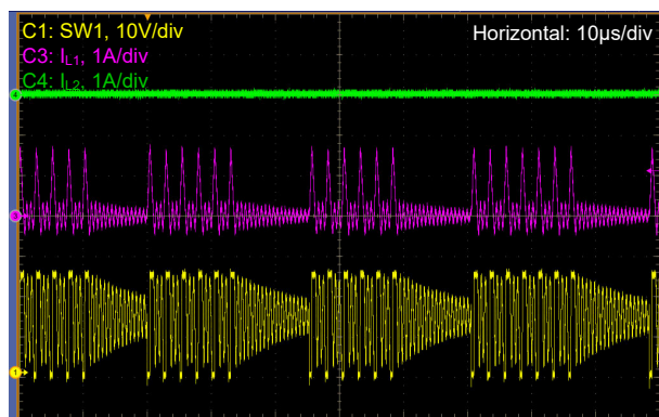
図 7-14. V_{in} = 14.4V 、 V_{out} = 24V 、DEM、 I_{load} = 0.1A
