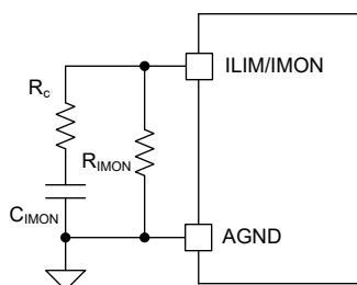
図 7-9. ILIM/IMON ピンの構成
