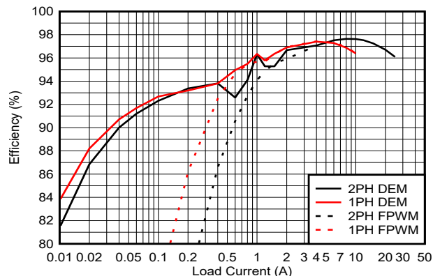
図 7-12. 効率と出力電流との関係、 V_{in} = 14.4V 、 V_{out} = 24V
