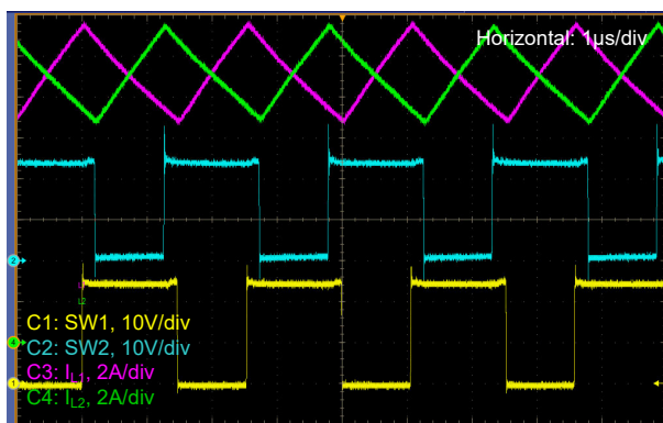
図 7-16. V_{in} = 14.4V 、 V_{out} = 24V 、DEM、 I_{load} = 15A
