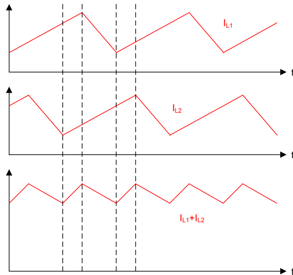
図 7-11. 正規化された出力コンデンサの RMS リップル電流
