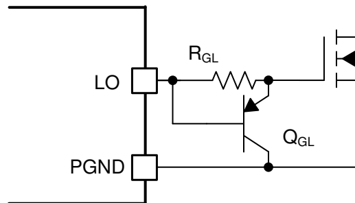
図 6-18. スルー レート制御
