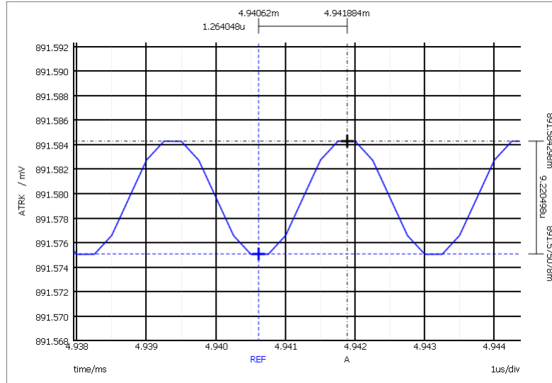
図 7-7. ATRK/DTRK の電圧リップル
