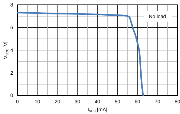
Figure 7. V_{VCC} と I_{VCC} との関係
