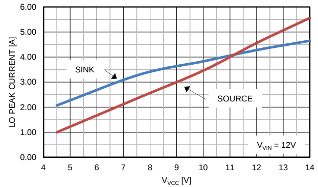
Figure 2. LOピーク電流と V_{VCC} との関係
