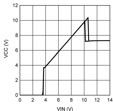
FIG 5-22. VCC vs VIN
