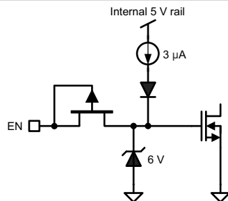
図 6-3. Enable Circuit
