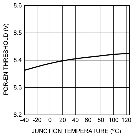
FIG 7-19. POR EN Threshold vs Temperature
