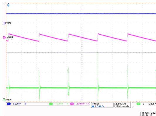
图 8-9. Light-Load Switching
