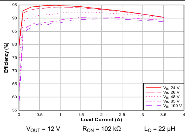
8-3. Conversion Efficiency (Linear Scale)
