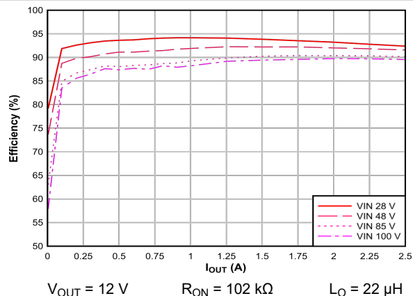
9-3. Conversion Efficiency (Linear Scale)
