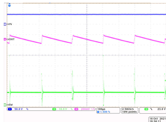
图 9-9. Light-Load Switching
