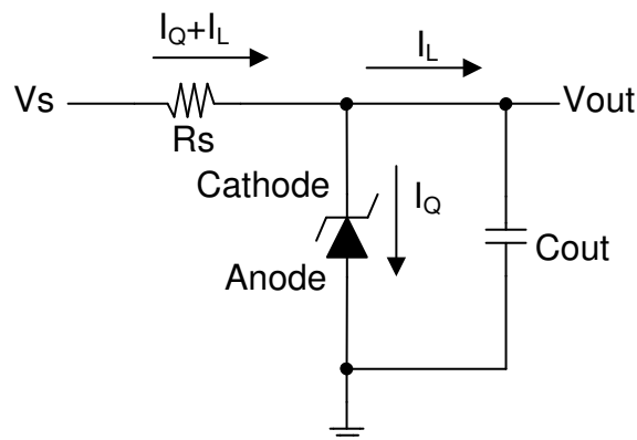
シャント レギュレータ回路図
