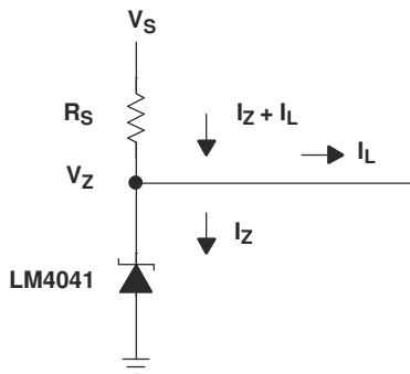
図 7-4. Shunt Regulator
