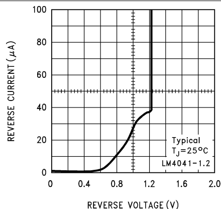
図 5-4. 逆方向特性と最小動作電流です
