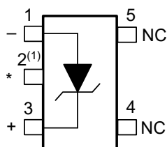
図 4-3. DCK パッケージ 5 ピン SC70 上面図
