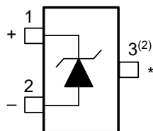
図 4-1. DBZ パッケージ 3 ピン SOT-23 上面図
