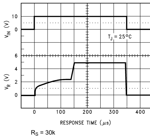
図 5-7. 入力電圧ステップ応答 LM4040-N-5
