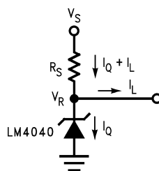
図 8-1. シェント レギュレータ回路図
