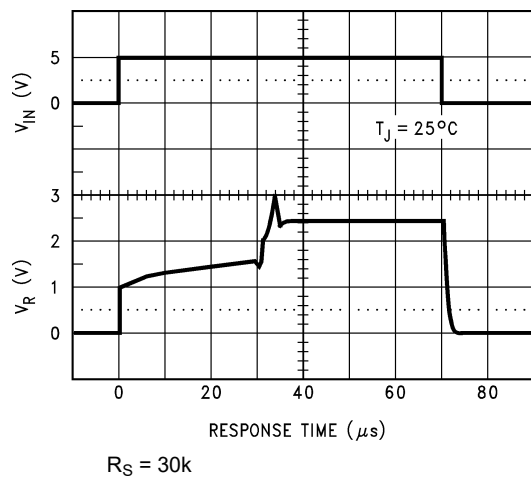
図 5-6. 入力電圧ステップ応答 LM4040-N-2.5
