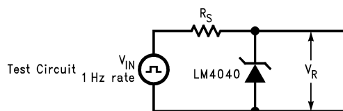
図 6-1. テスト回路
