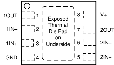
図 4-1. D、DGK、JG、P、PS、DDF、PW パッケージ 8 ピン SOIC、VSSOP、PDIP、SO、TSSOP 上面図
