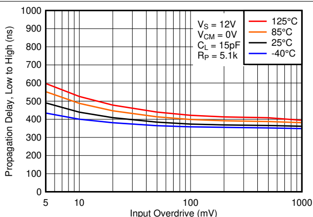
図 5-28. Low から High までの伝搬遅延と入力オーバードライブ電圧との関係、12V
