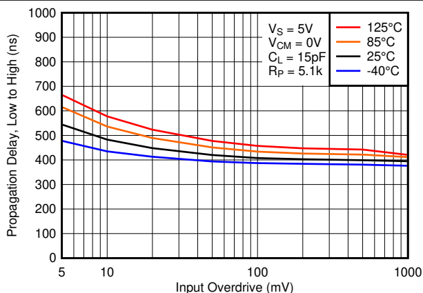
図 5-26. Low から High までの伝搬遅延と入力オーバードライブ電圧との関係、5V
