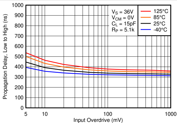
図 5-30. Low から High までの伝搬遅延と入力オーバードライブ電圧との関係、36V
