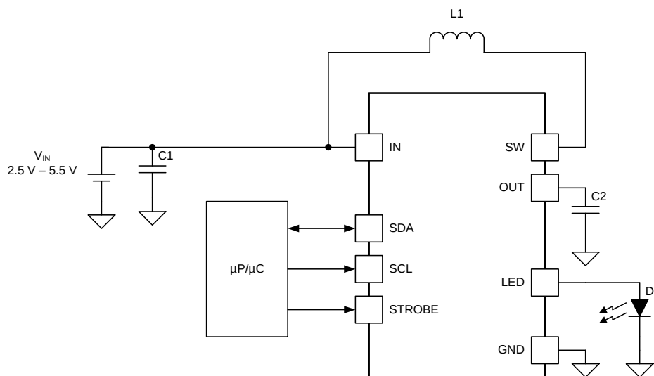
概略回路図
