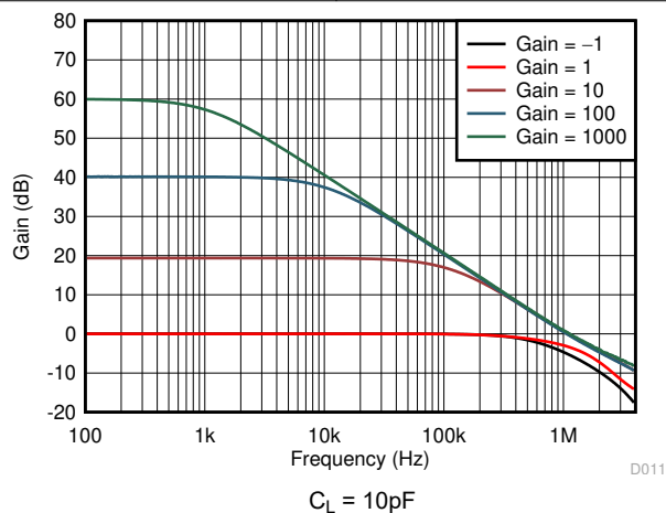
図 6-5. 閉ループ・ゲインと周波数との関係
