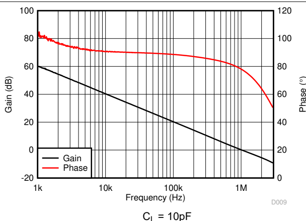
図 6-3. 開ループ・ゲインおよび位相と周波数との関係
