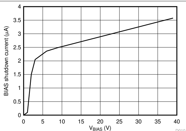
7-10. I_{\text{SHUTDOWN(BIAS)}} vs V_{\text{BIAS}}
