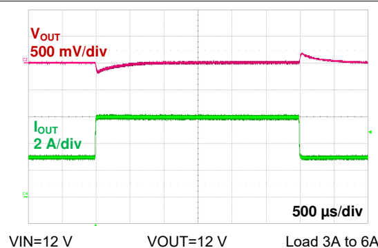
6-16. Load Step (Buck-Boost)
