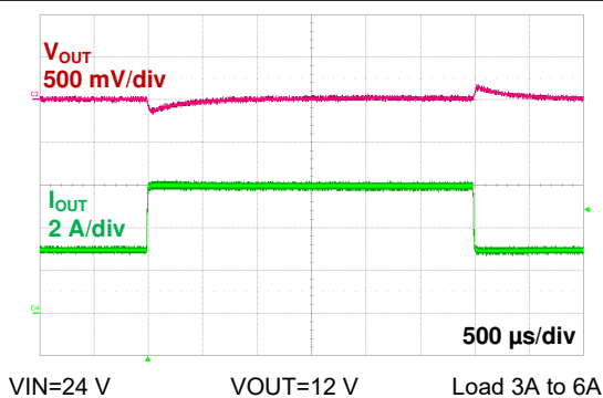
6-17. Load Step (Buck)
