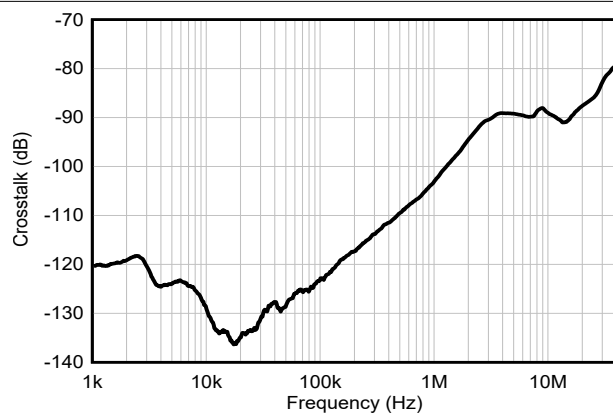
図 5-33. チャネル セパレーションと周波数との関係
