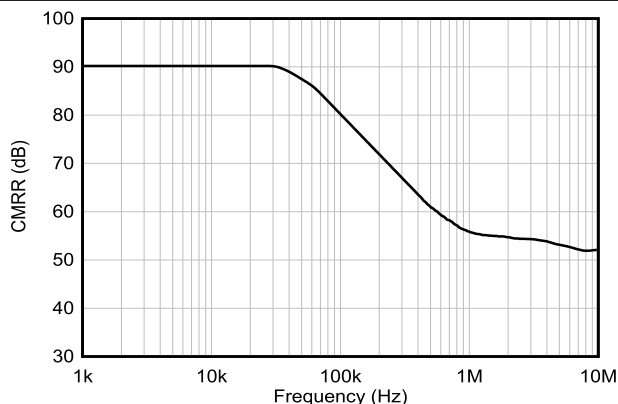
図 5-8. CMRR と周波数との関係
