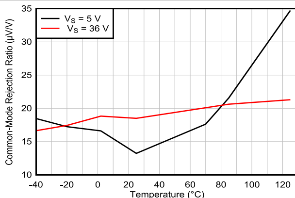
図 5-10. 同相除去比と温度との関係
