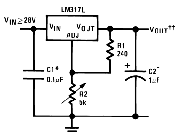
回路図
