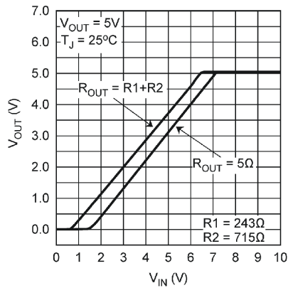
図 6-7. Line Regulation (Legacy Chip)
