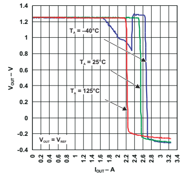
図 6-2. Load Regulation (Legacy Chip)
