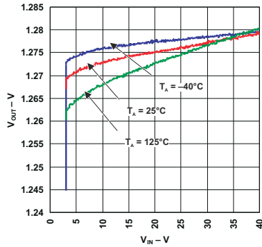
図 6-7. Line Regulation (Legacy Chip)
