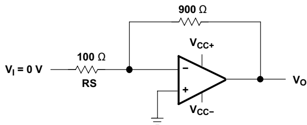
図 8-2. ノイズ・テスト回路
