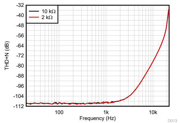
図 7-18. THD+N 比と周波数との関係、 G = 1 G = 1 、 f = 1\text{kHz} 、 BW = 80\text{kHz} 、 V_{OUT} = 10\text{V}_{PP} 、 R_L を V_- に接続
