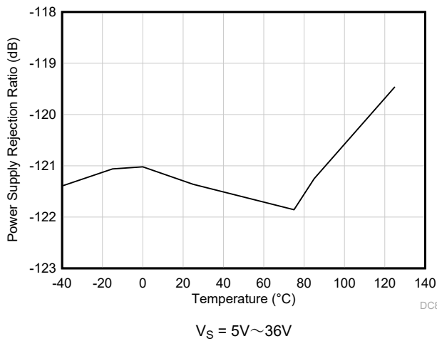
図 7-15. 電源除去比と温度との関係 (dB)
