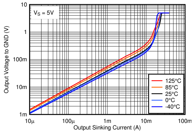
図 5-20. 出力 Low 電圧と出力シンク電流の関係、5V
