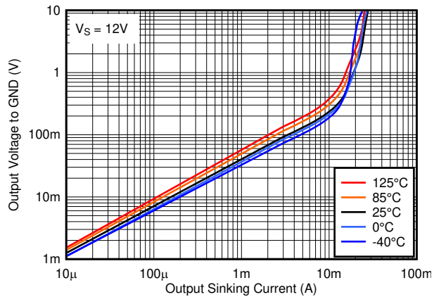
図 5-21. 出力 Low 電圧と出力シンク電流の関係、12V
