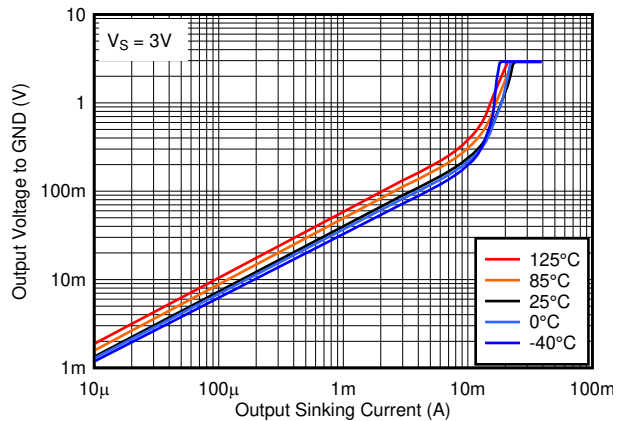
図 5-19. 出力 Low 電圧と出力シンク電流の関係、3V
