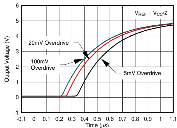
図 5-32. 各種オーバードライブの応答時間、Low から High への遷移
