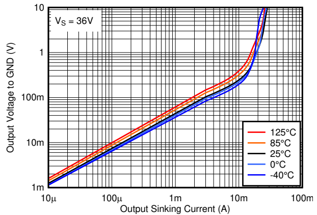
図 5-22. 出力 Low 電圧と出力シンク電流との関係、36V
