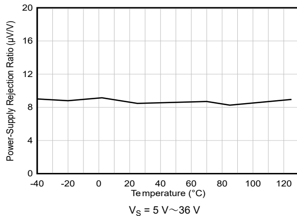
図 5-11. 電源除去比と温度との関係
