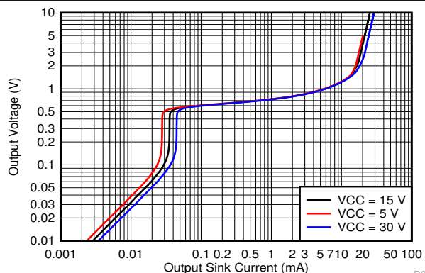
図 5-35. 出力シンク特性
