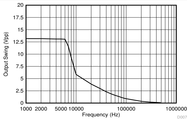
図 5-40. 最大出力スイングと周波数との関係 (VCC = 15V)
