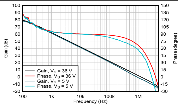
図 5-5. 開ループゲインおよび位相と周波数との関係
