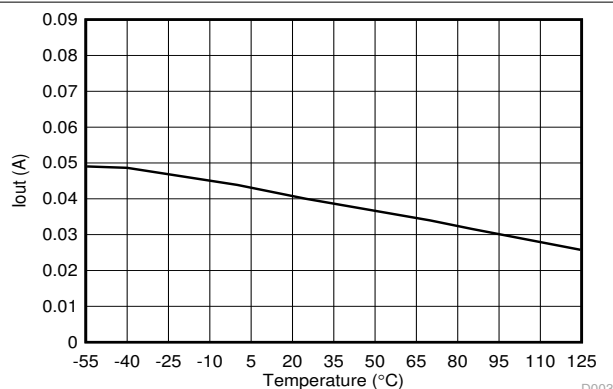
図 5-37. ソース電流制限
