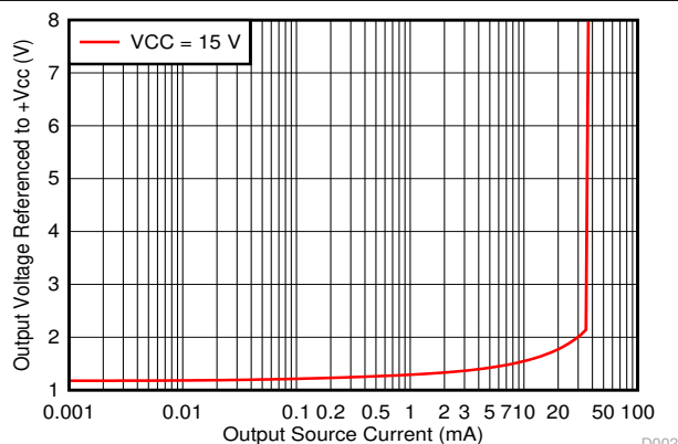
図 5-36. 出力ソース特性
