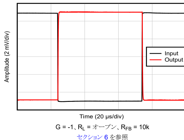
図 5-27. 小信号ステップ応答, G = -1
