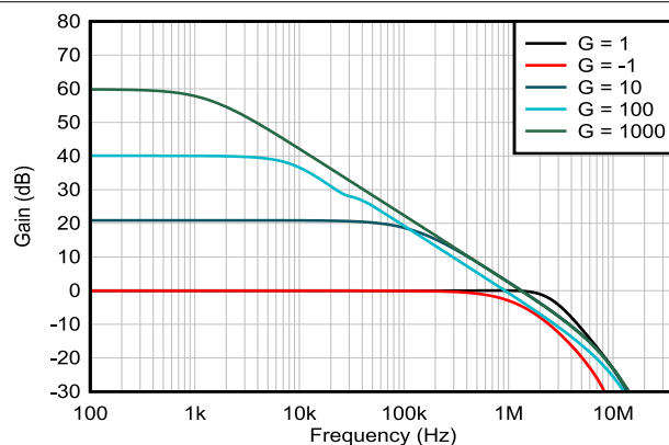
図 5-6. 閉ループゲインと周波数との関係
