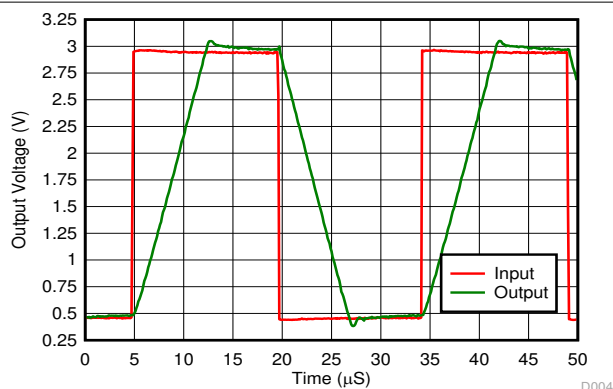
図 5-38. 電圧フォロワの大信号応答 (50pF)
