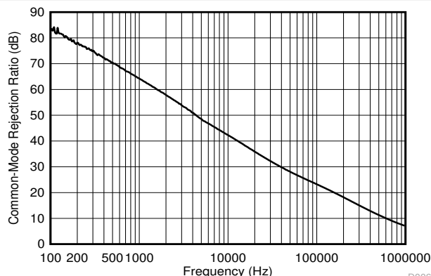
図 5-39. 同相除去比
